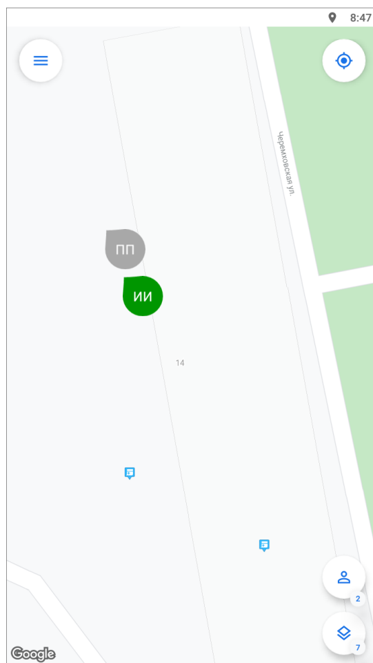
Рис. 2.67: Окно «Карта»
