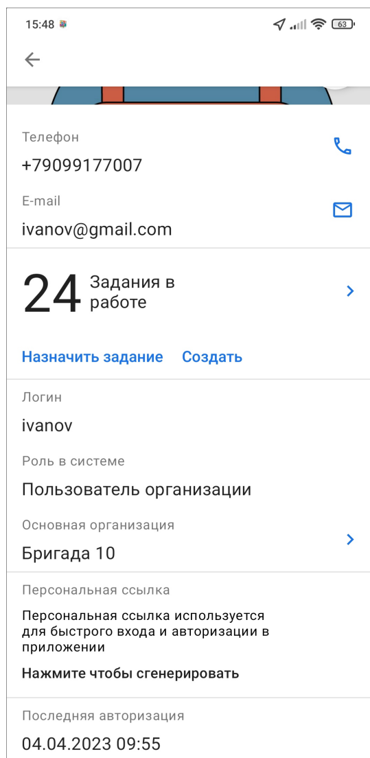
Рис. 2.43: Профиль пользователя
