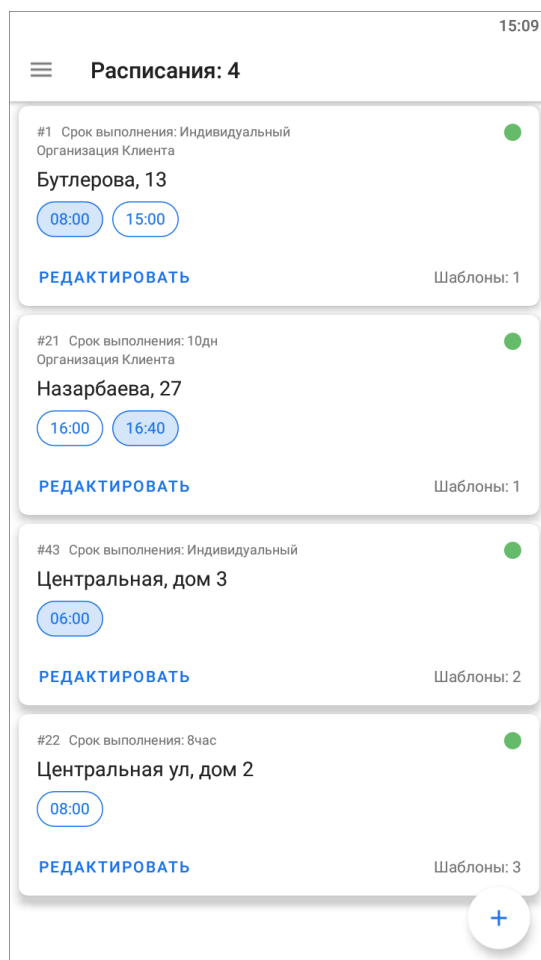
Рис. 2.80: Список расписаний
