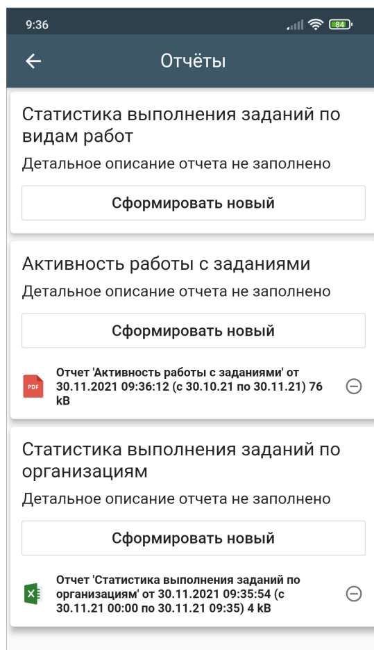
Рис. 2.82: Окно «Отчеты»
