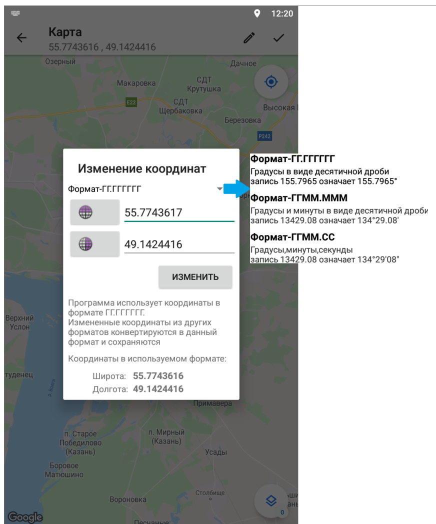
Рис. 2.30: Изменение координат
