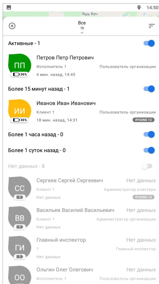
Рис. 2.71: Окно «Пользователи»
