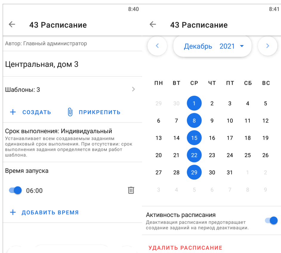
Рис. 2.79: Создание расписания
