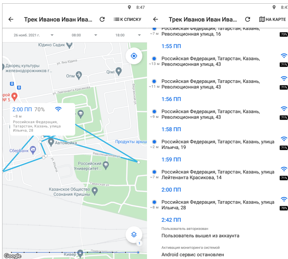
Рис. 2.73: Просмотр трека
